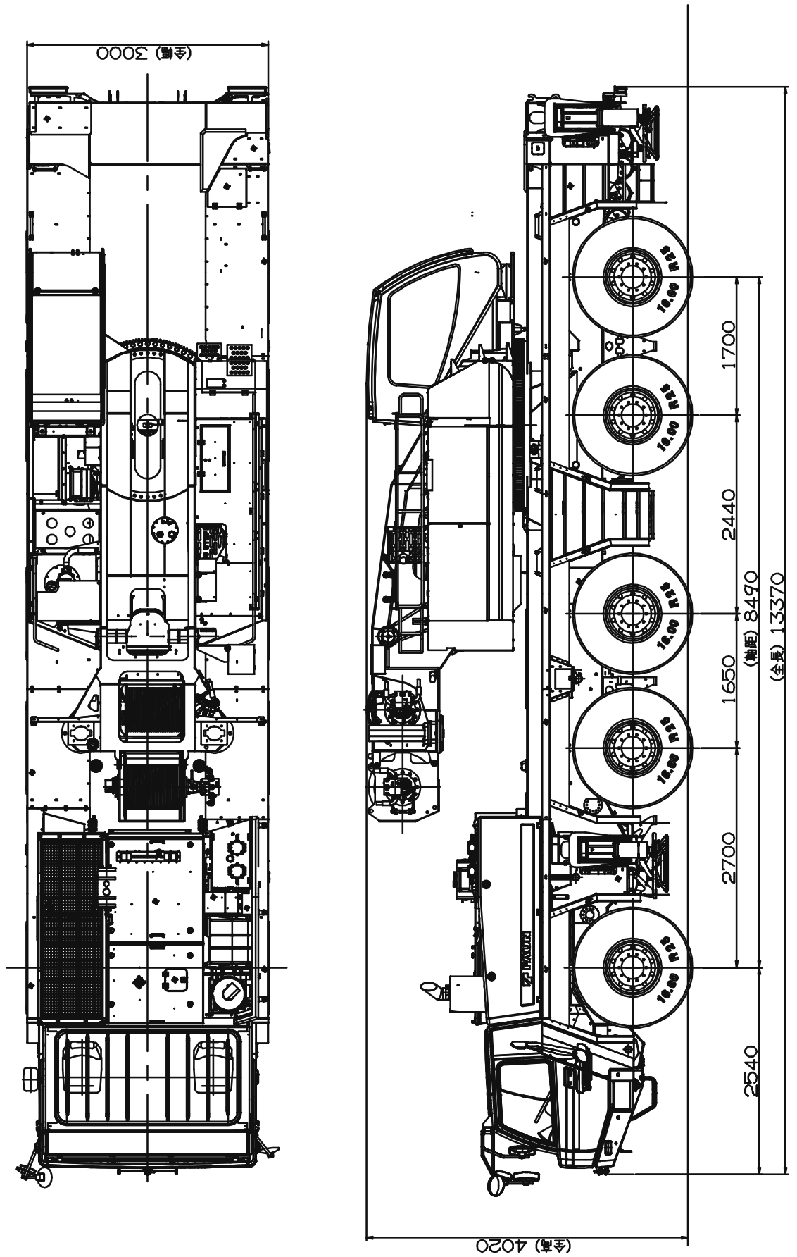
4. 外觀圖 [ 公道走行狀態 ]
